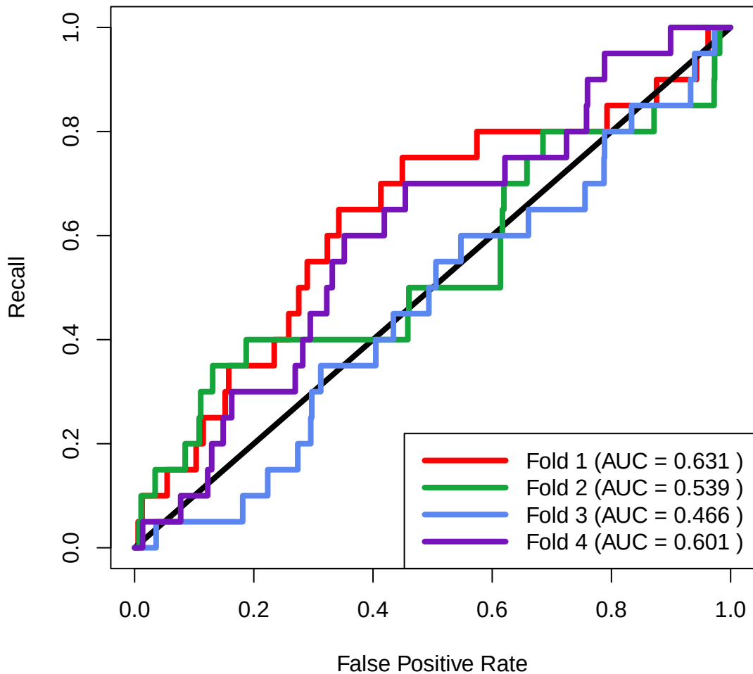
Primig 2000 Dataset 3: 24x20x8x1 Validation
